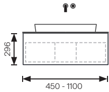
PLI01 1 Ladenelement (Siphon-Lade)*
