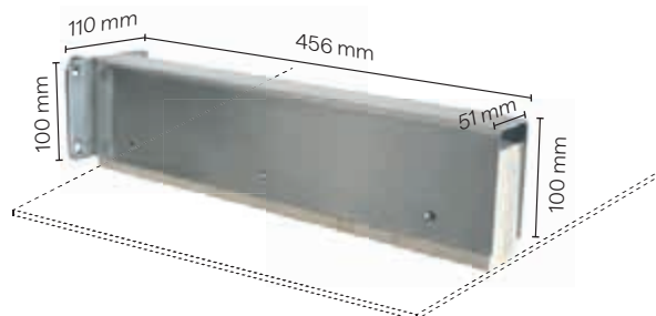
KT02 Konsolenträger mit verstellbarer Holzeinlage
