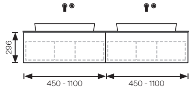
PLI02 2 Ladenelemente (Siphon-Laden)*
