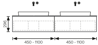
PLI02 2 Ladenelemente (Siphon-Laden)*
